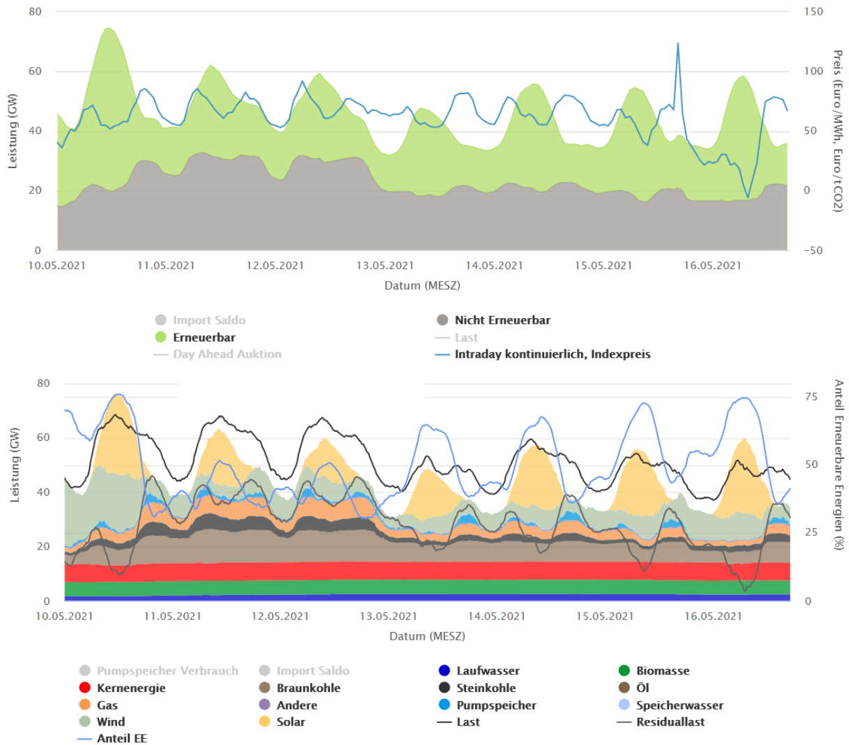
Abbildung 23: Beispiel für den Verlauf von Börsenstrompreisen, konventioneller und regenerativer Stromerzeugung der 19. Kalenderwoche im Mai 2021 [ISE4].
