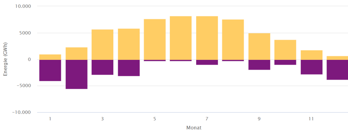
Abbildung 12: Nettostromimport (violett) und Solarstromproduktion (gelb) im Jahr 2022 für Deutschland [ISE4].
