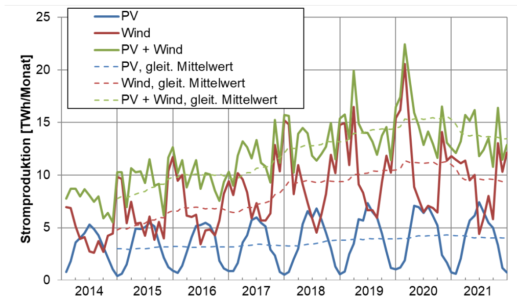
Abbildung 22: Monatssummen PV- und Windstromproduktion, Daten aus [ISE4].
