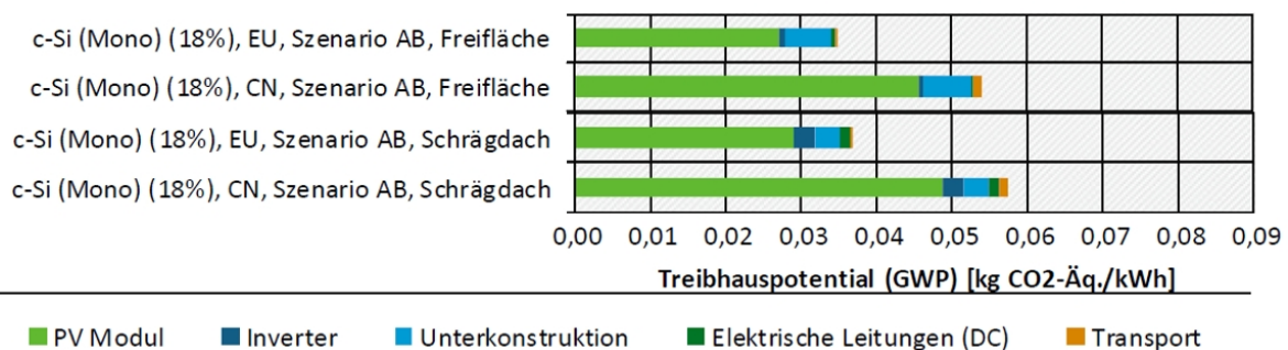
Abbildung 40: Treibhauspotenzial der Stromerzeugung mit mono c-Si PV für Dach- und Freiflächenanlagen [UBA7].
