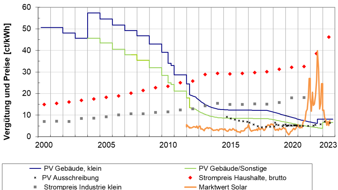
Abbildung 6: Feste EEG-Einspeisevergütung für PV-Strom nach dem Datum der Inbetriebnahme des Kraftwerks in aktuelle Anlagenklassen „Gebäudeanlagen mit Überschusseinspeisung bis 10 kW p “ und „Sonstige Anlagen bis 100 kW“ aus [Netz2] und [BNA3], mittlere Vergütung in den Ausschreibungen der Bundesnetzagentur [BNA3], Strompreise [BMWK1], [BDEW1] mit Schätzung für 2023, Marktwert Solarstrom [NETZ1].
