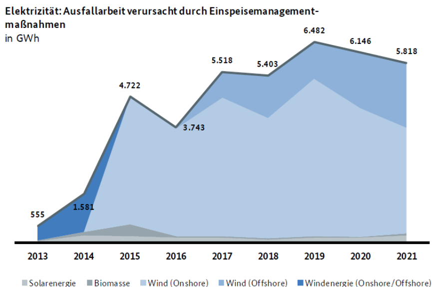
Abbildung 19: Abgeregelte elektrische Energie [BNA2].
