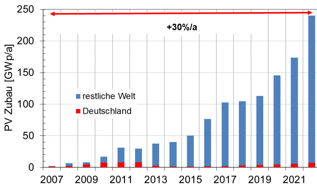
Abbildung 43: Entwicklung des jährlichen PV-Zubaus [IEA3] und mittlere jährliche Wachstumsrate.
